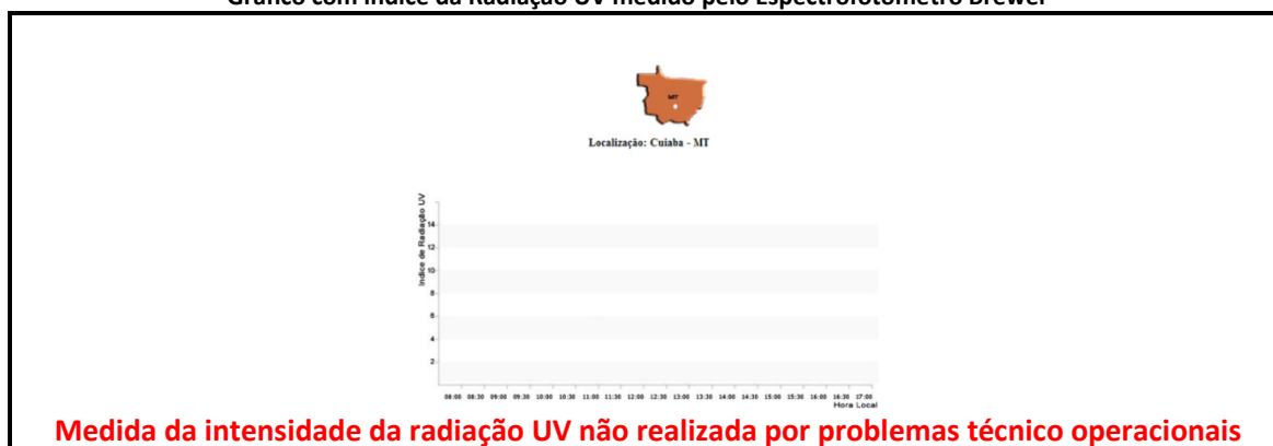
Gráfico com índice da Radiação UV medido pelo Espectrofotômetro Brewer
